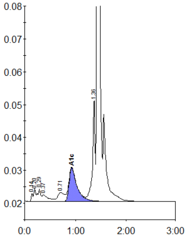
Peak table - ID: 10514562
